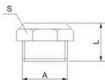
■ 外观图/overall Dimension
