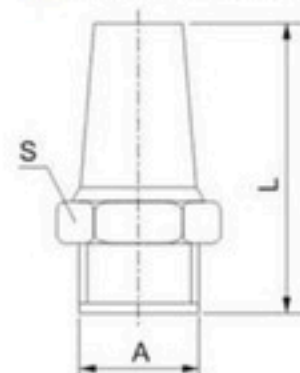
■ 外观图/overall Dimension
