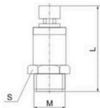
■ 外观图/overall Dimension
